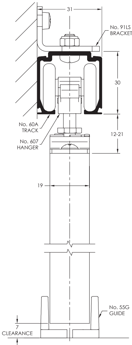
91LS BRACKETS
